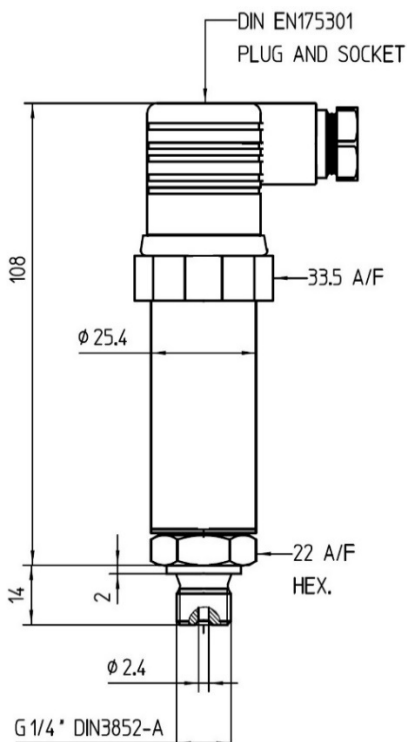
DIN Connection
